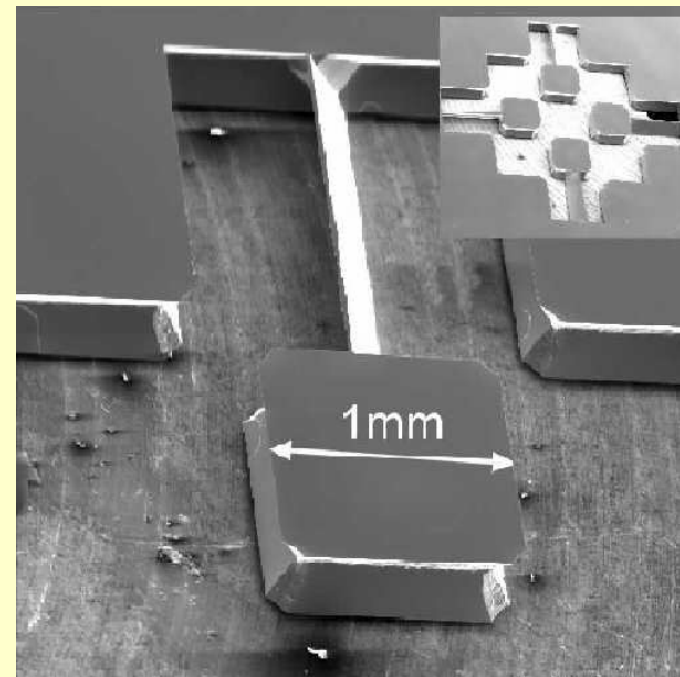
Beschleunigungssensor
