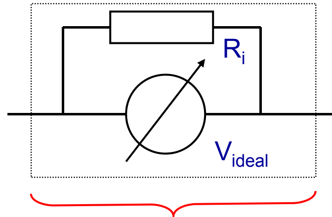
reales Voltmeter
