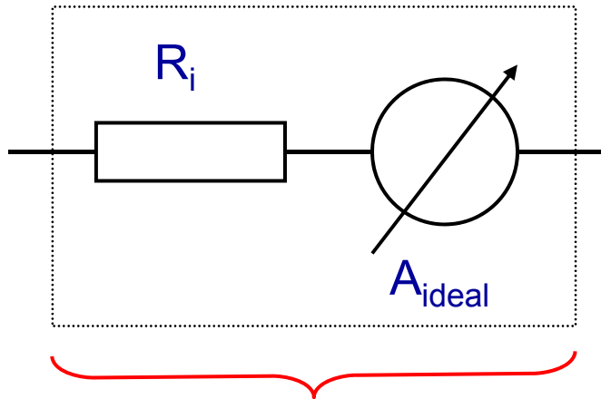
reales Ampèremeter
