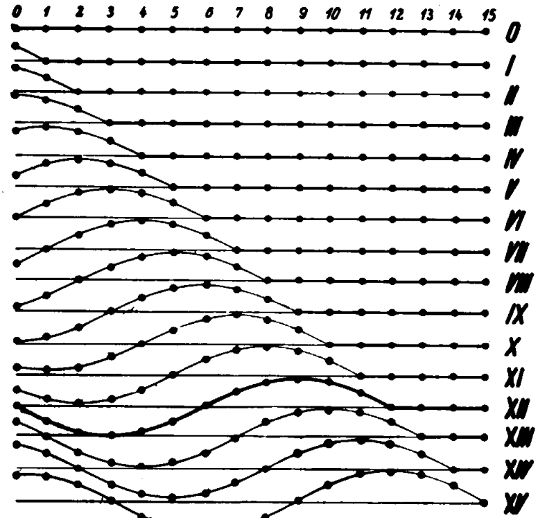
Abb. 420. Bildung einer fortschreitenden T
