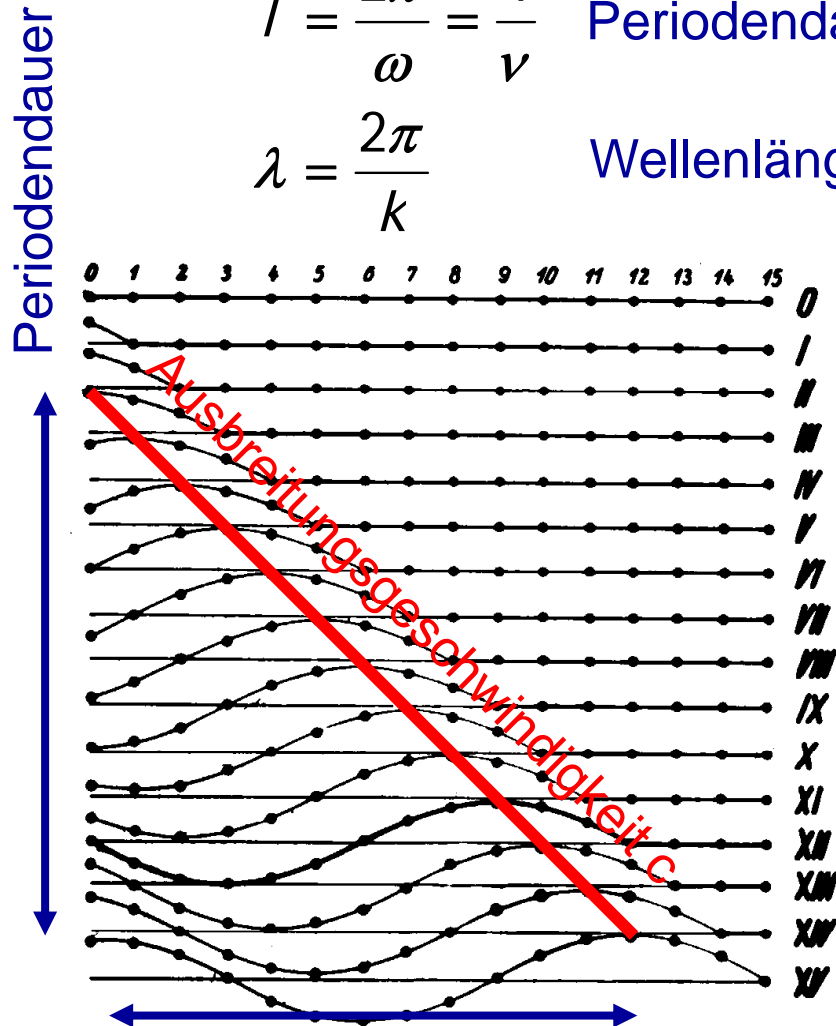
Abb. 430. Bildung einer fortschreitenden Welle
