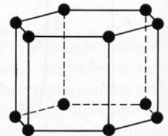
hexagonales Gitter
